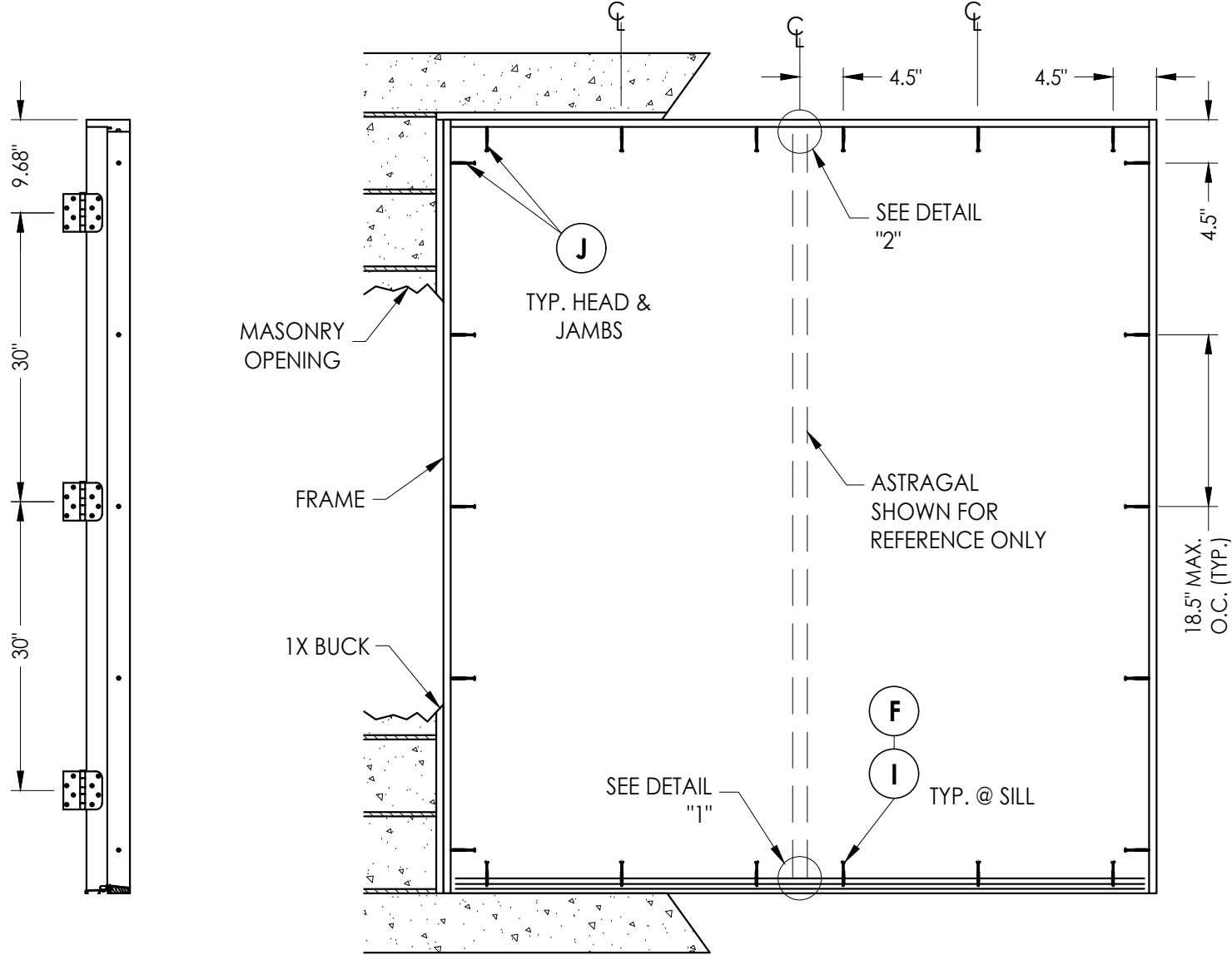
HINGE JAMB
